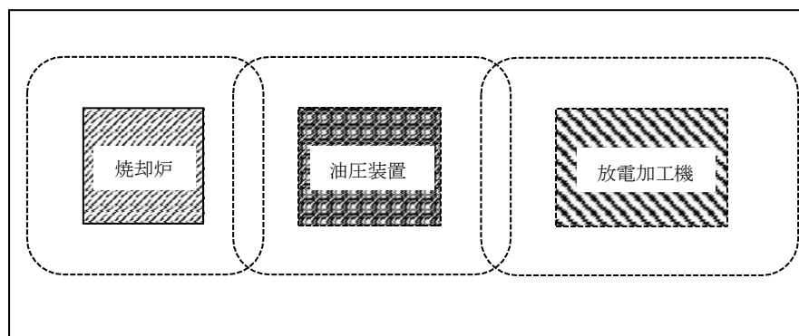
第8-6図 部分規制の一般取扱所と認めることができない例
