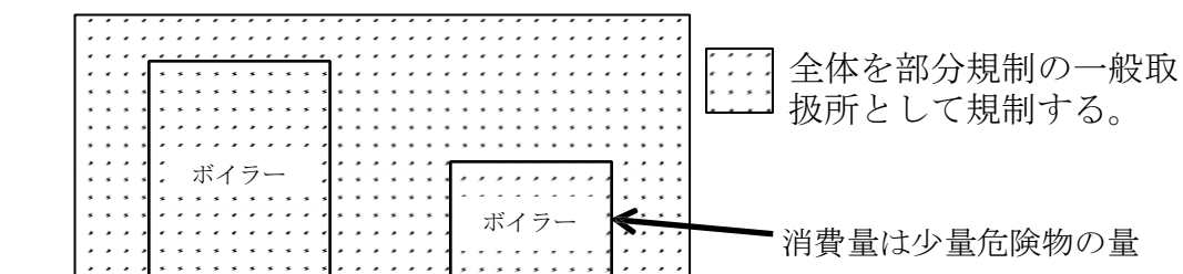
第8－11図 全体を一般取扱所とした例
