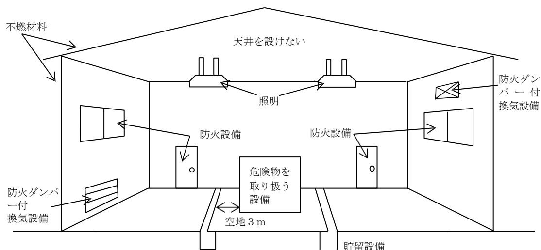
第 8－16 図 一般取扱所の例
