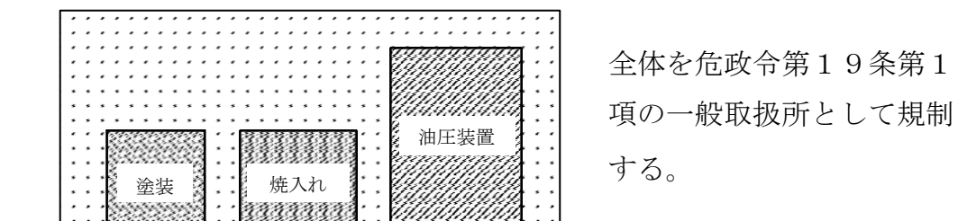
第8-5図 部分規制の一般取扱所とすることができない例
